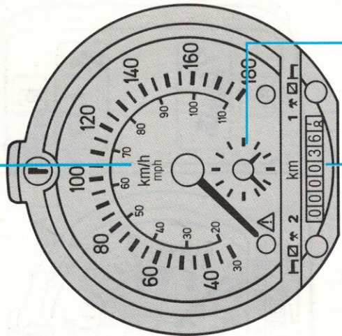
Indicateur de vitesse
