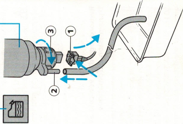
Capteur de présence d'eau du filtre à gazole
