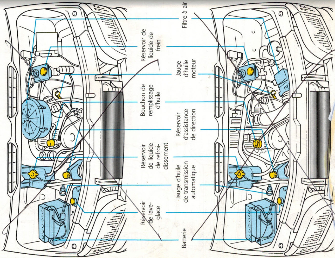
Compartment moteur - moteur 2,0 litres ACT à carburateur
