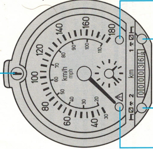
Bouton de sélection 2ème conducteur
