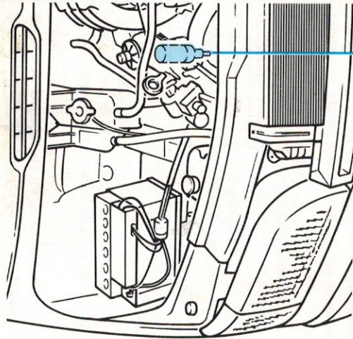
Capteur de présence d'eau du filtre à gazole
