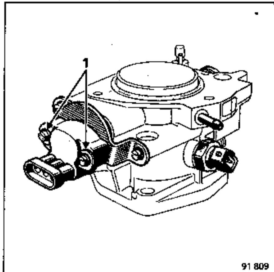
MOTEUR Z7W
