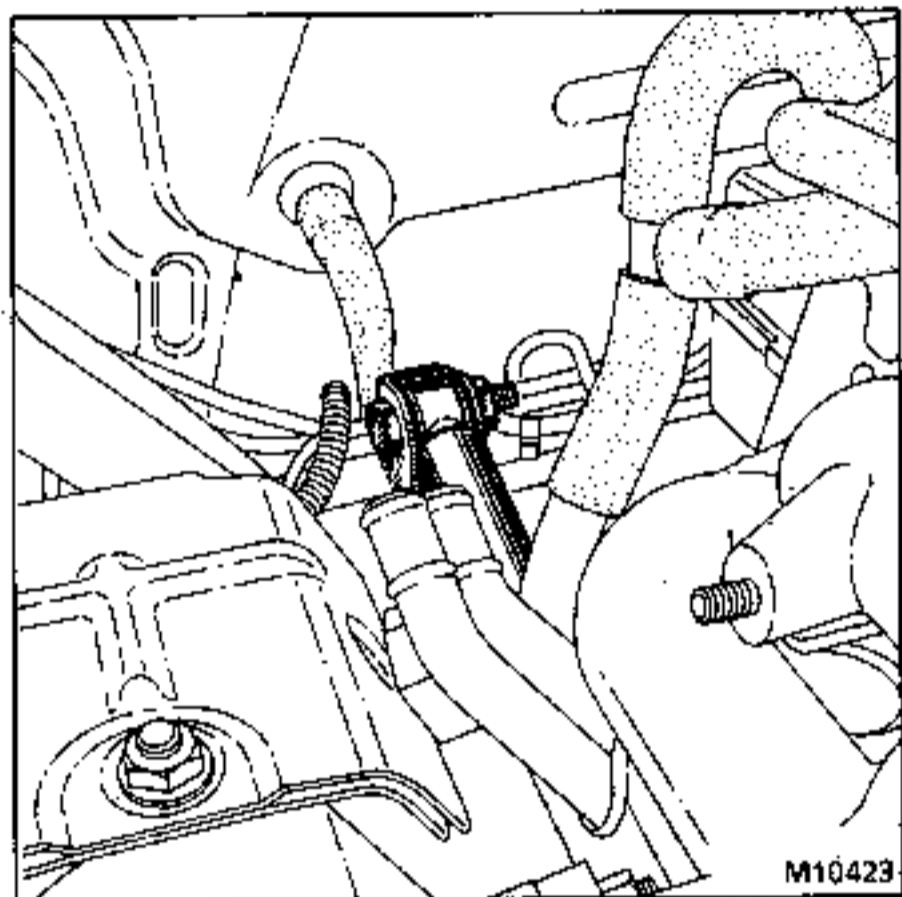
(MOTEUR J8S)
