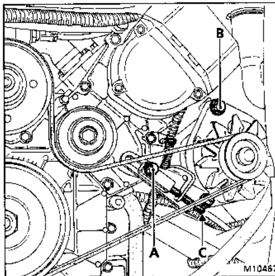
MOTEUR Z7W
